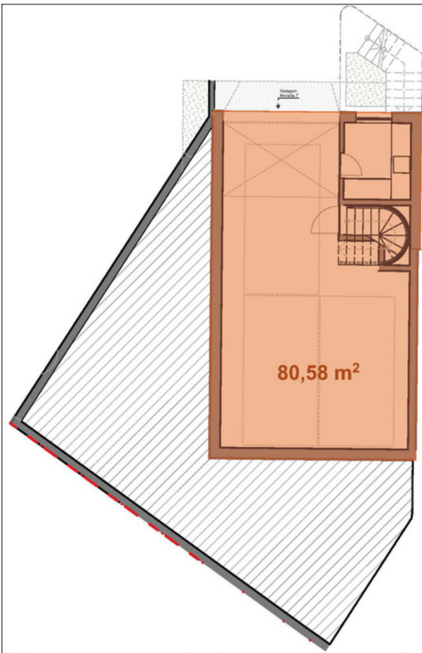
01. Piso Cave 1:150
