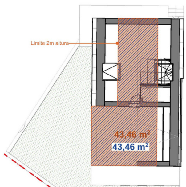
04. Piso Sótão 1:150
