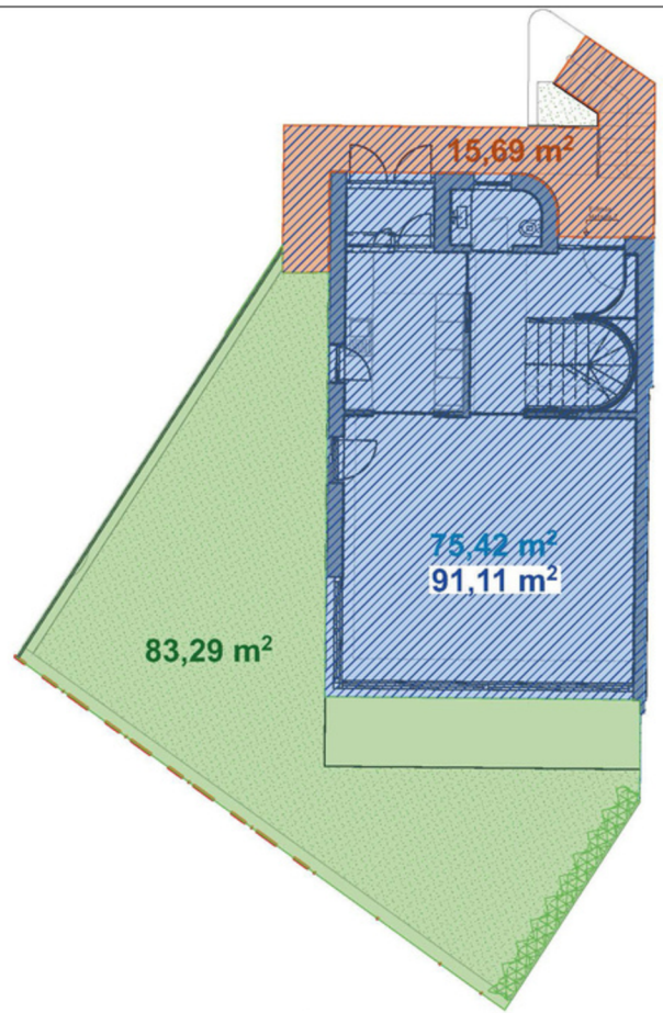
02. Piso 00 1:150
